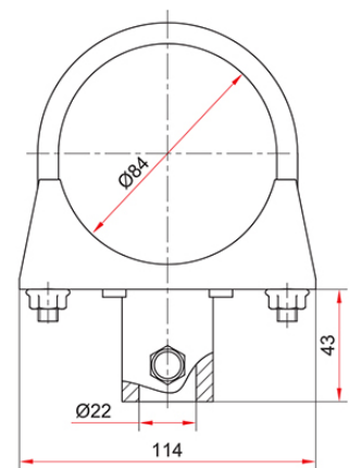
Кронштейн для ТМД-4-421Р
